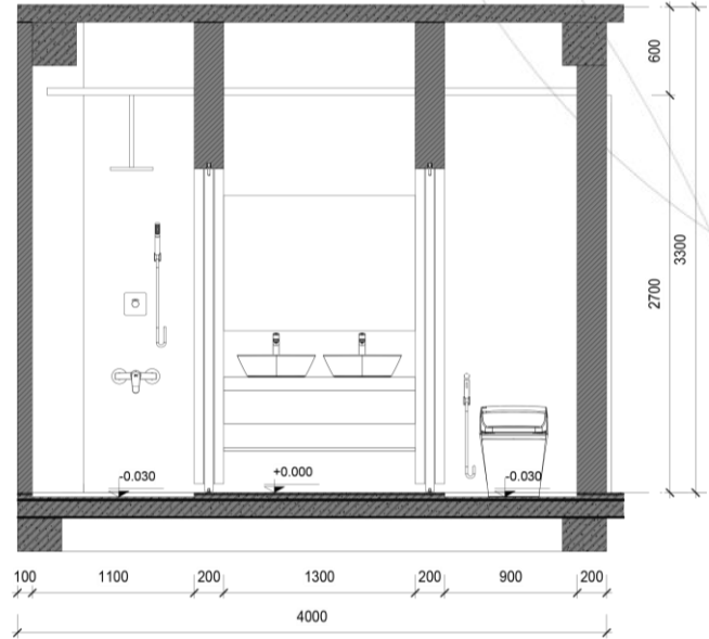
ELEVATION
