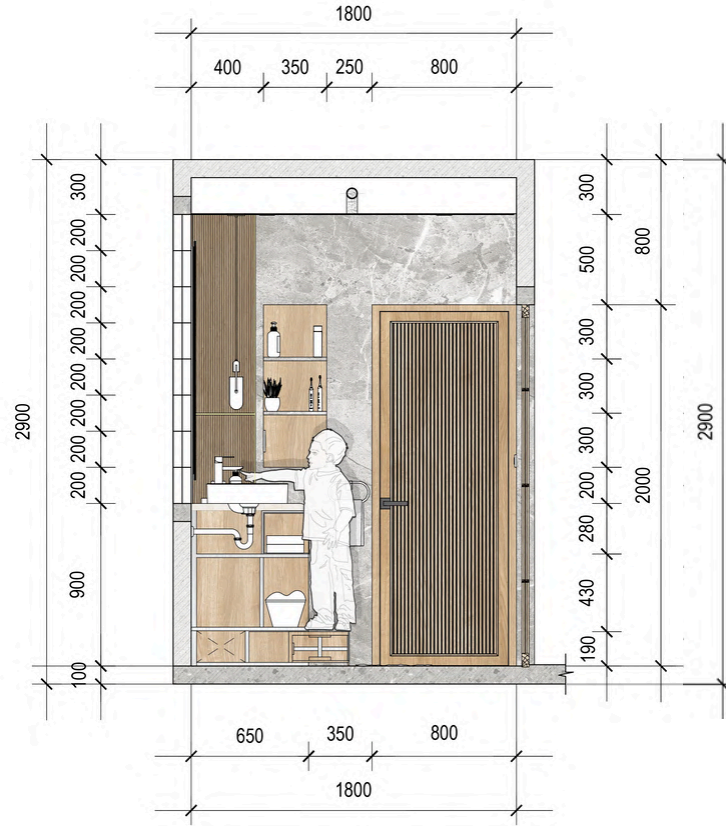
ELEVATION B-B
