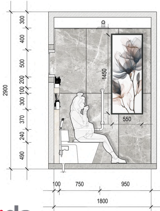
SECTION TOILET
