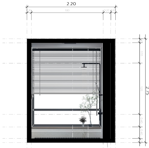
Elevation 3
