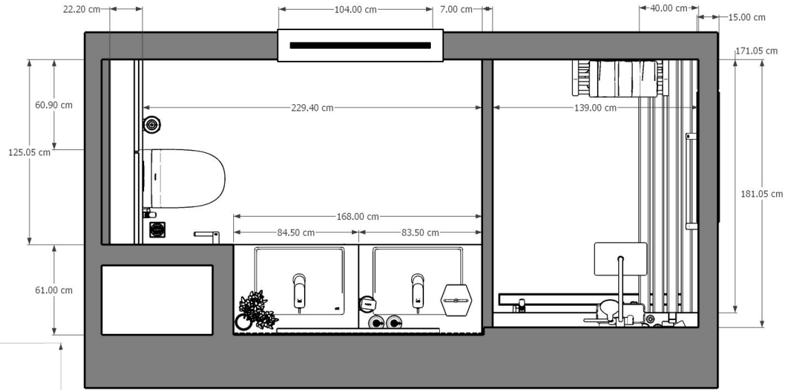
Top Elevation
