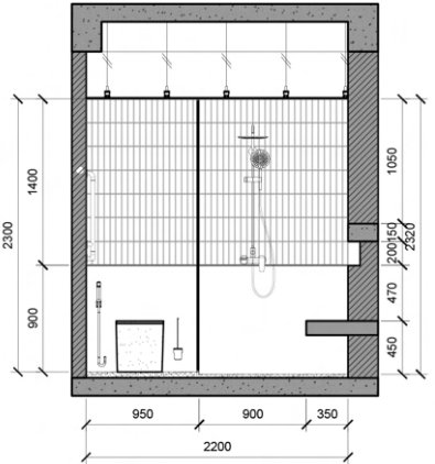
ELEVATION B
