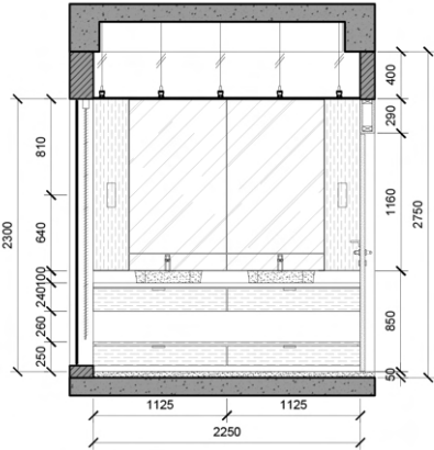
ELEVATION A
