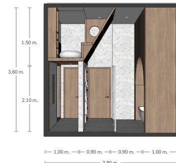
Elevation 4
