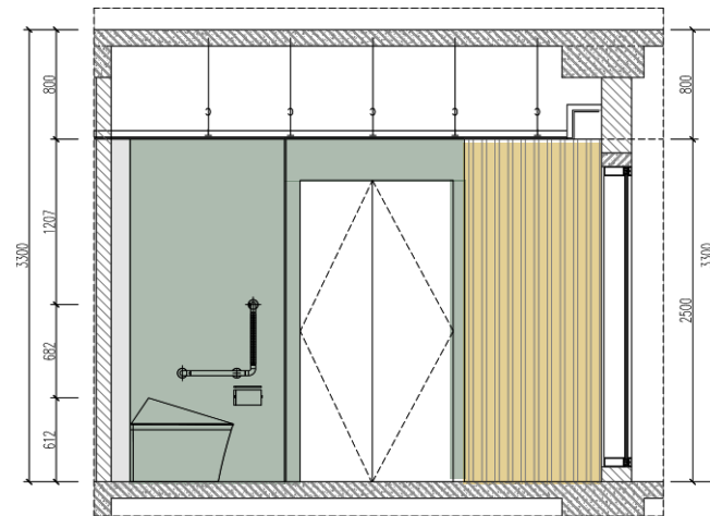
MẶT ĐỨNG 3
